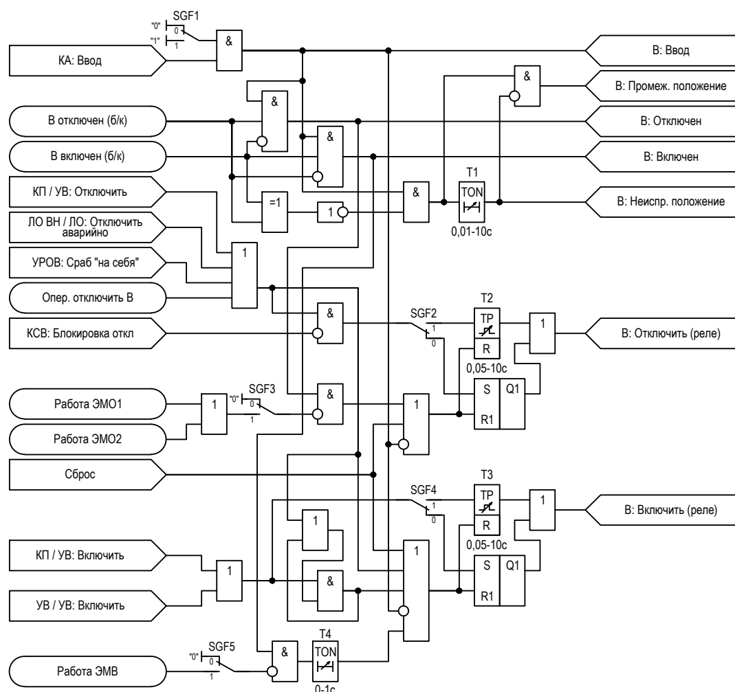
Рисунок 2.33 – Функциональная схема логики выключателя
