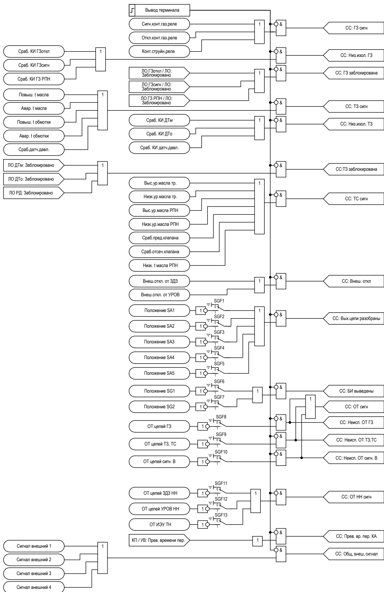
Рисунок 2.34 – Функциональная схема логики сборки сигналов
