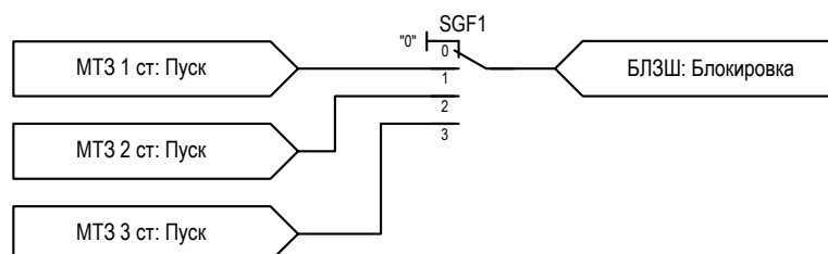
Рисунок 2.3 – Функциональная схема логики БЛЗШ
