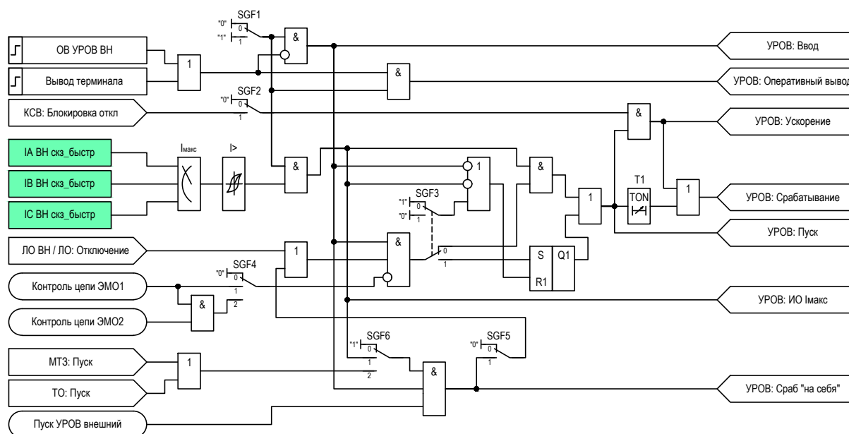
Рисунок 2.26 – Функциональная схема логики УРОВ
