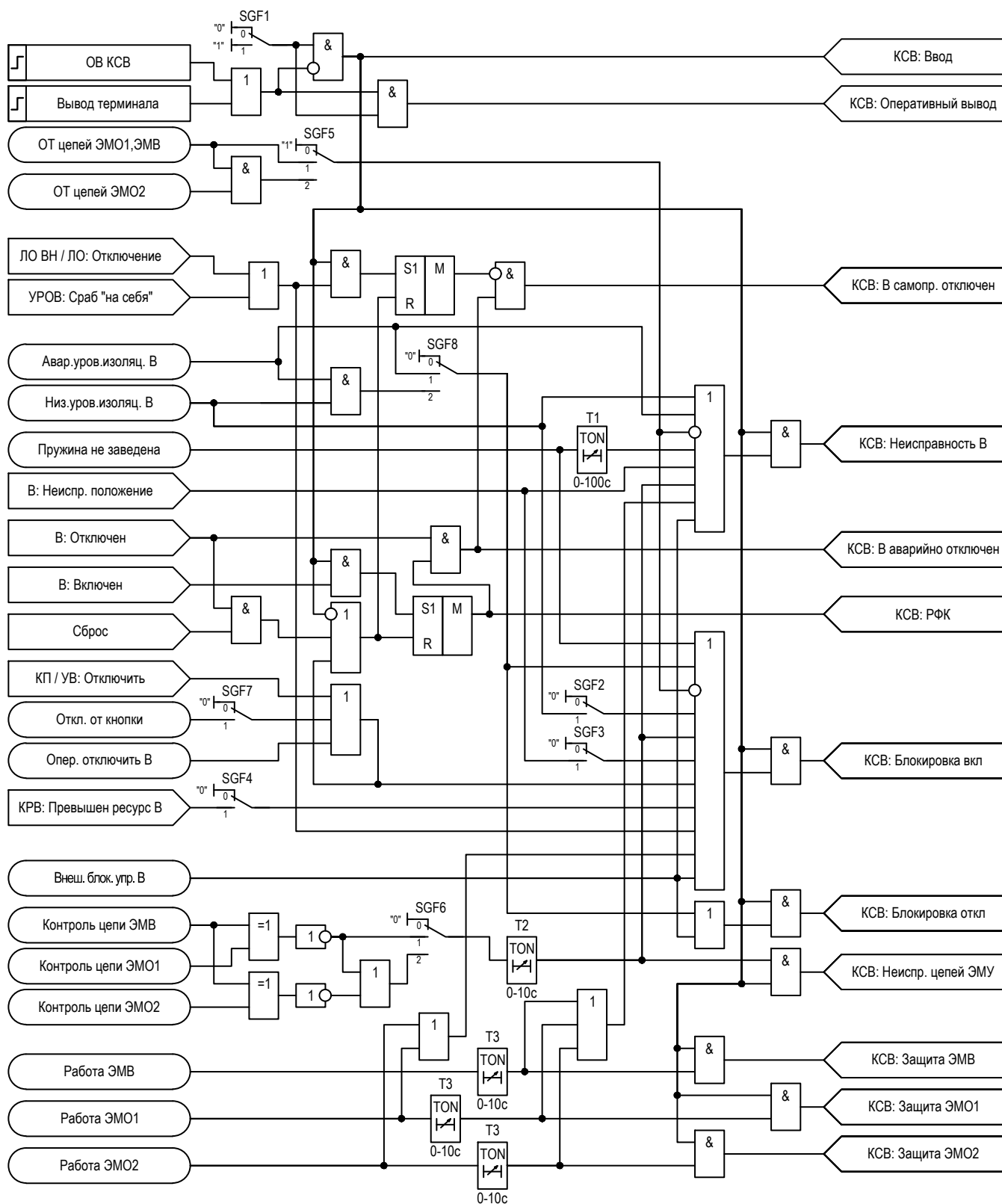
Рисунок 2.28 – Функциональная схема логики КСВ
