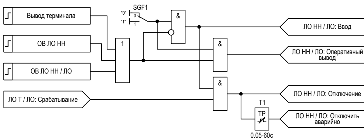
Рисунок 2.23 – Функциональная схема логики отключения выключателя
