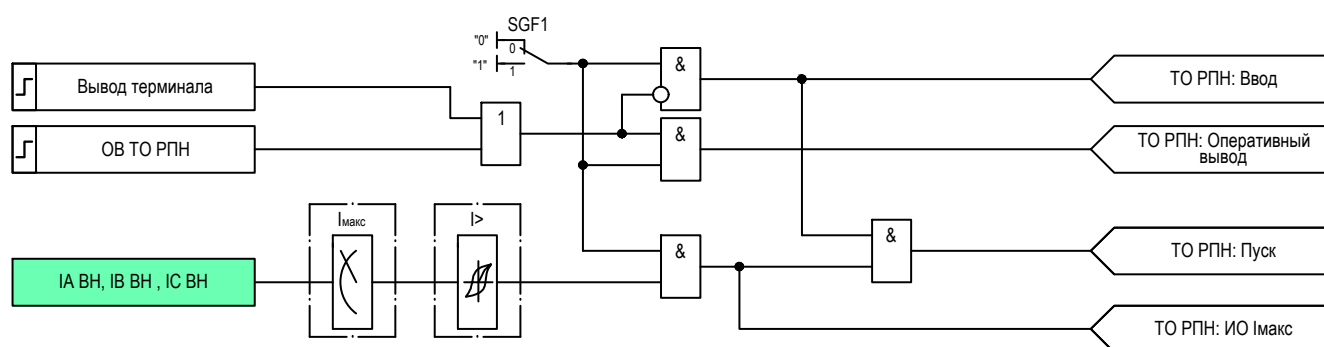
Рисунок 2.10 – Функциональная схема логики ТО РПН
