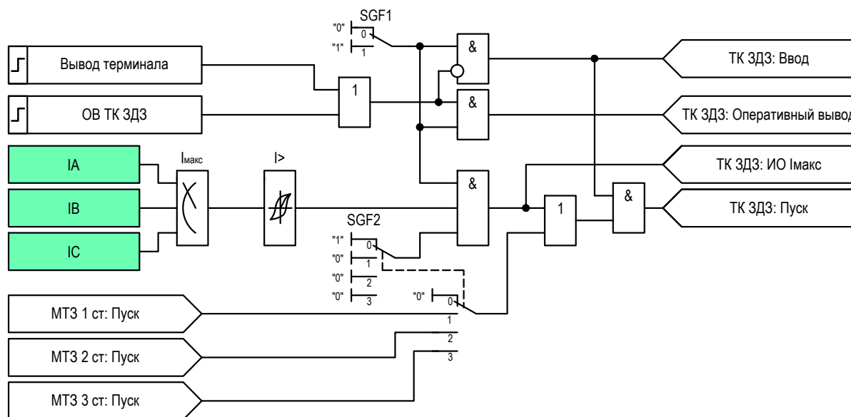
Рисунок 2.9 – Функциональная схема логики ТК ЗДЗ
