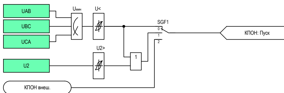
Рисунок 2.2 – Функциональная схема логики КПОН
