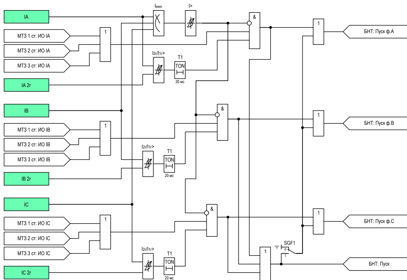
Рисунок 2.4 – Функциональная схема логики БНТ
