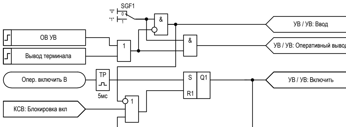
Рисунок 2.31 – Функциональная схема логики УВ
